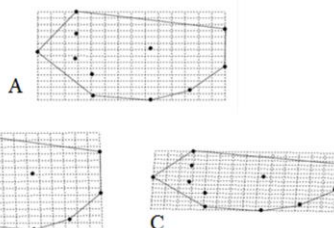
شکل ۶. (A) شکل بال (جلویی) مرجع در محور RW1، (B) شکل بال در حد نهایی منفی محور RW1 (مربوط به جمعیت پسیل معمولی پسته از استان کرمان) و (C) شکل بال در حد نهایی مثبت محور RW1 (مربوط به جمعیت‌های پسیل معمولی پسته از استان خراسان رضوی)
