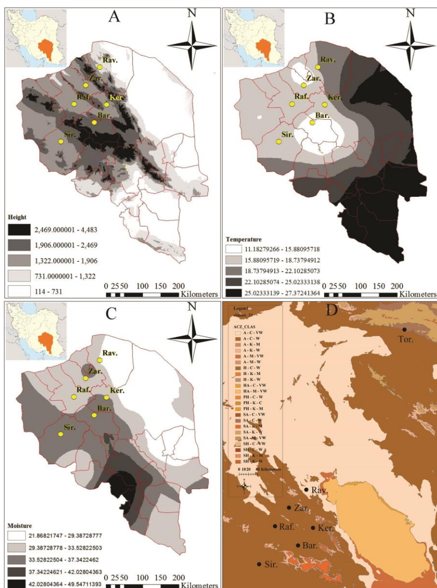
شکل ۲. نقشه توپوگرافی (A)، دمایی (B)، رطوبتی (C) و اقلیمی (D) نقاط گردآوری جمعیت‌های مختلف جغرافیایی پسیل معمولی پسته در
