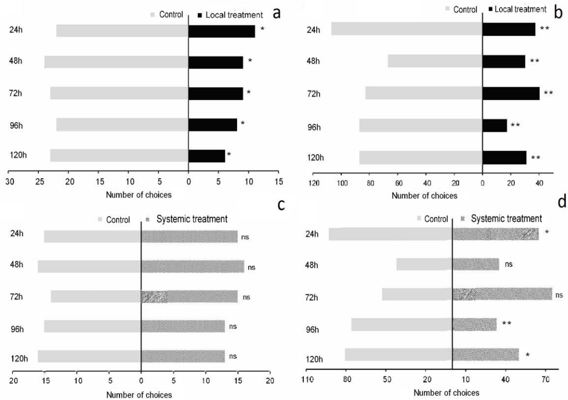
شکل ۳. پراکنش افراد بالغ شسته پنبه Aphis gossypii در آزمایش ترجیح دو انتخابی بین شاهد و تیمار موضعی (a) و بین شاهد و تیمار سیستمیک (c) روی گیاهان آسیب دیده توسط افراد هم گونه در بازه زمانی بین ۲۴ تا ۱۲۰ ساعت. پراکنش پوره های شسته پنبه Aphis gossypii در آزمایش ترجیح دو انتخابی بین شاهد و تیمار موضعی (b) و بین شاهد و تیمار سیستمیک (d) روی گیاهان آسیب دیده توسط افراد هم گونه. ستاره ها بیانگر تفاوت معنی دار بین دو گروه است.
