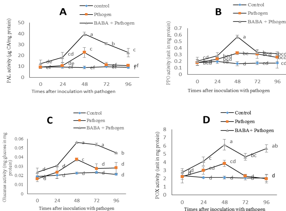
شکل ۳. میزان فعالیت آنزیم فنیل الانین آمونیا لیاز (A)، پلی فنل کسیداز (B)، گلوکاناز (C) و پراکسیداز (D) در گیاهان خیار در فاصله‌های زمانی مختلف پس از تلقیح با P. cubensis ، دادها با روش تجزیه واریانس تحلیل و مقایسه میانگین‌ها با آزمون توکی انجام شد. تیمارهای دارای حرف‌های مشترک اختلاف معنی‌داری ندارند ( P \leq 0.05 ).
